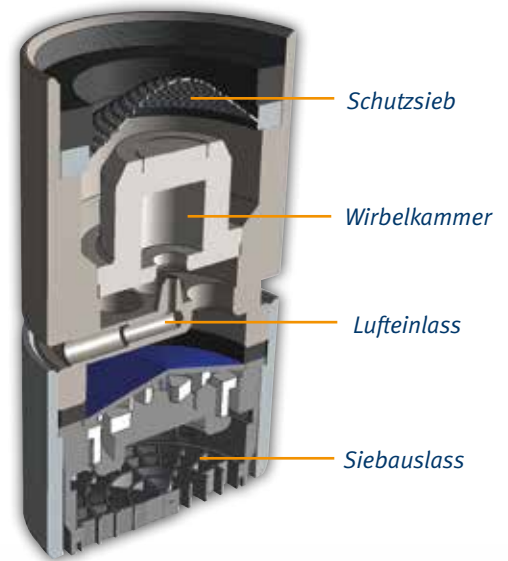
Querschnitt eines ECO-Wirblers
