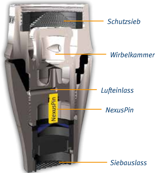
Querschnitt eines VITA-Wirblers
